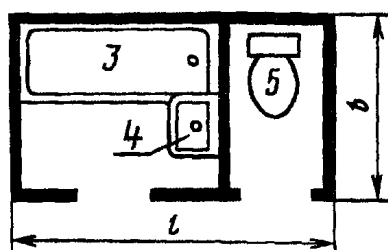
Левые варианты исполнения кабин
