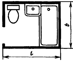
Тип 4СК
