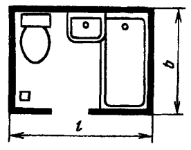
Тип 5СК
